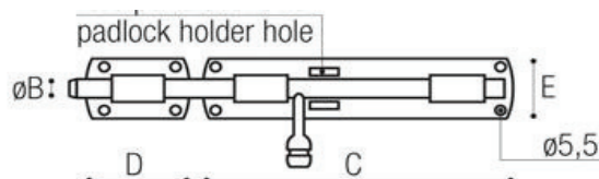
ALI248 INOX P/LUCCHETTO L100/150
