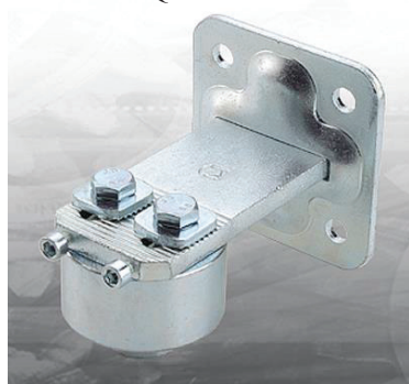
A CUSCINETTO C/PIASTRA D70 BI345RGPST
