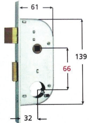
2 MANDATE+SCROCCO CILINDRO D26 MG.149.32.0
