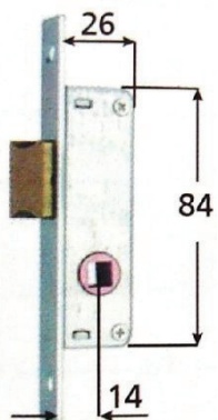
SOLO SCROCCO FRONTALE L20 MG.901.14.2
