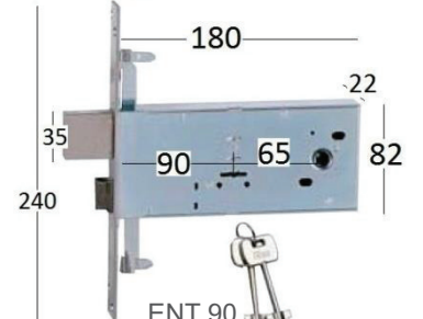
ENT. 90 C/SCROCCO 3 PUNTI ISE983901 BFZ
