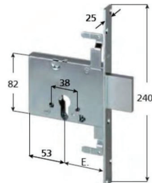
FASCIA E=70 CIL. EU 3 PUNTI CIS56016.70
