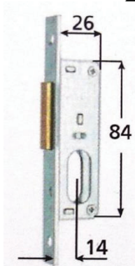
1 MANDATA CIL. OVALE MG.906.14.2
