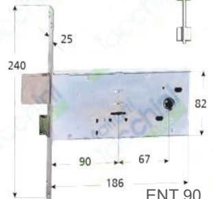
ENT. 90 CON SCROCCO ISE981901 BFZ
