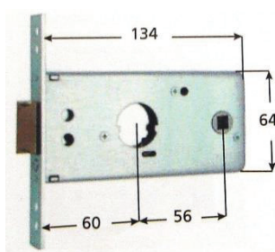
1 MAND.+SCROCCO CILINDRO D22 MG.288.60.2
