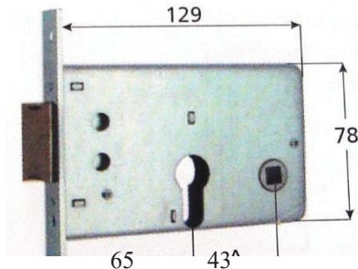
1 MAND.+SCROCCO CILINDRO EU MG.312.65.2
