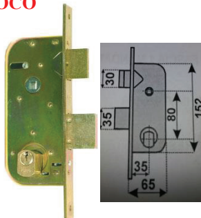
2 MAND.+SCROCCO CIL. OVALOIDE ISE620350
