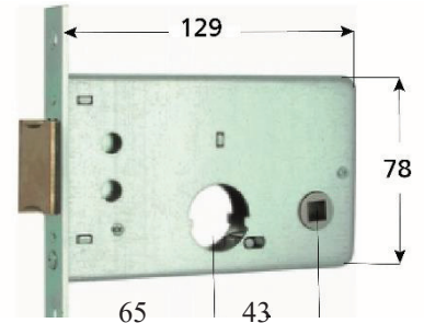
1 MAND.+SCROCCO CILINDRO D22 MG.313.65.2
